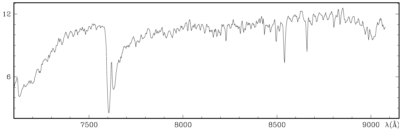
Fig. 92. ESO 1.5m + B&C spectrum of ER Del
